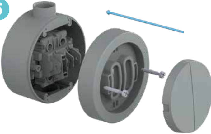
Contayı belirtilen yönde çekerek yuvasından çıkartın
