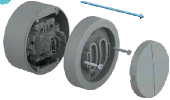
Kapak ve montaj vidalarını çıkarın
