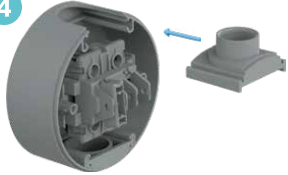
Conta yuvasına boru contasını yerleştirin
